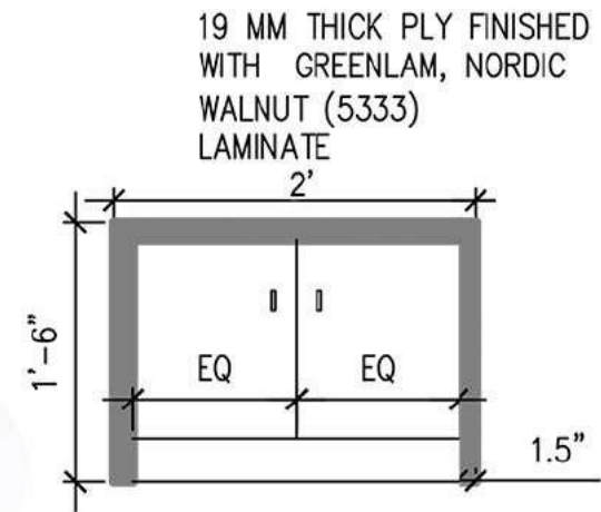
2 ELEVATION Scale: 1:50
